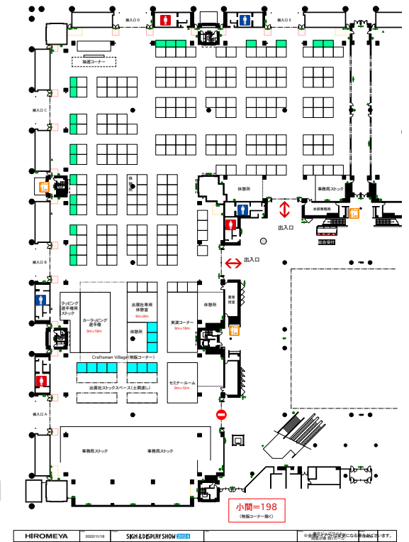
参考平面図
